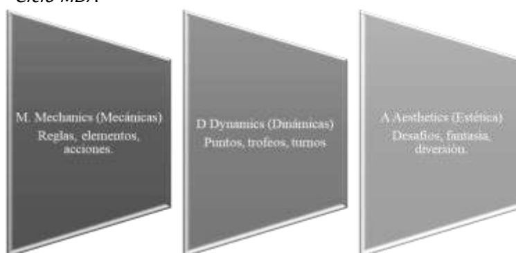
Figura1 Ciclo MDA
